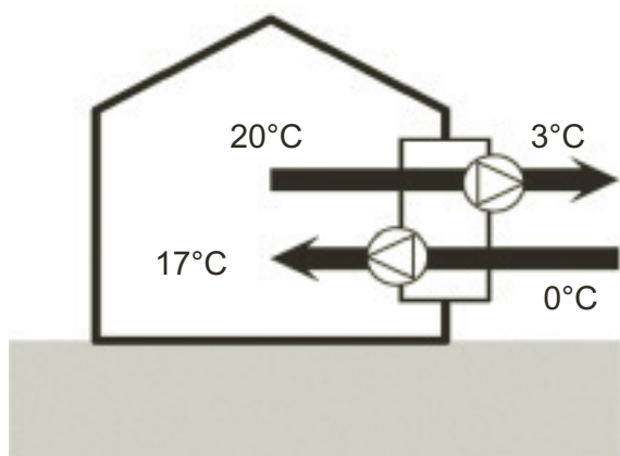
WTW (wintersituatie)
