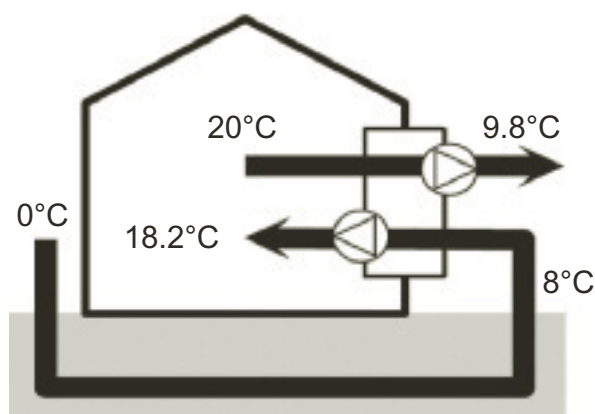
bodemluchtWTW (wintersituatie)
